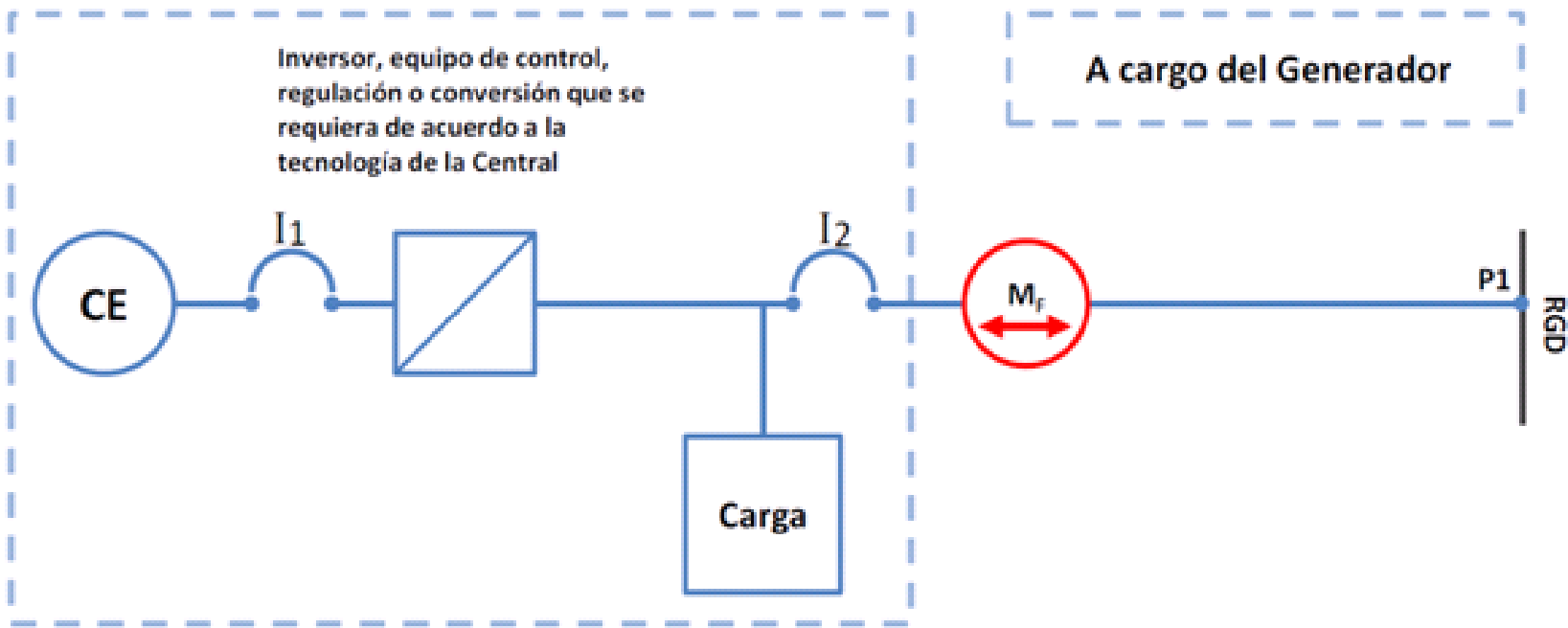
Esquema de interconexión 2 para Centrales Eléctricas menores o iguales que 250 kW en Media Tensión con Centros de Carga.
