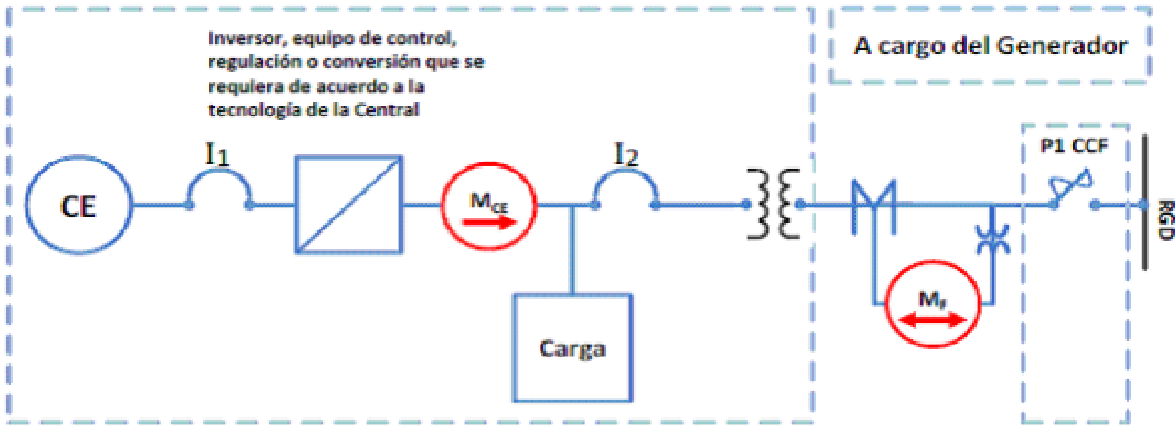
Esquema de interconexión 7 para Centrales Eléctricas menores o iguales que 50 kW en Baja Tensión.
