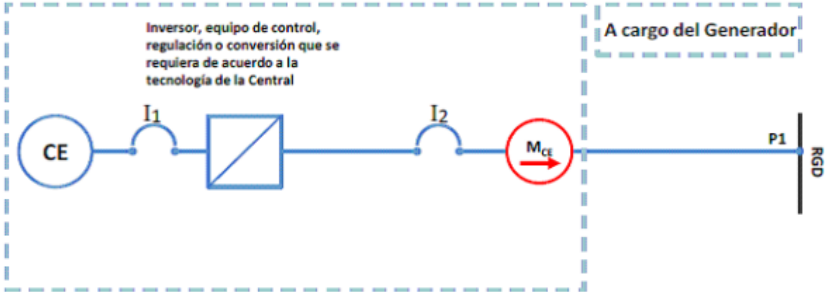
Esquema de interconexión 8 para Centrales Eléctricas menores o iguales que 250 kW en Media Tensión con medición en Baja Tensión.
