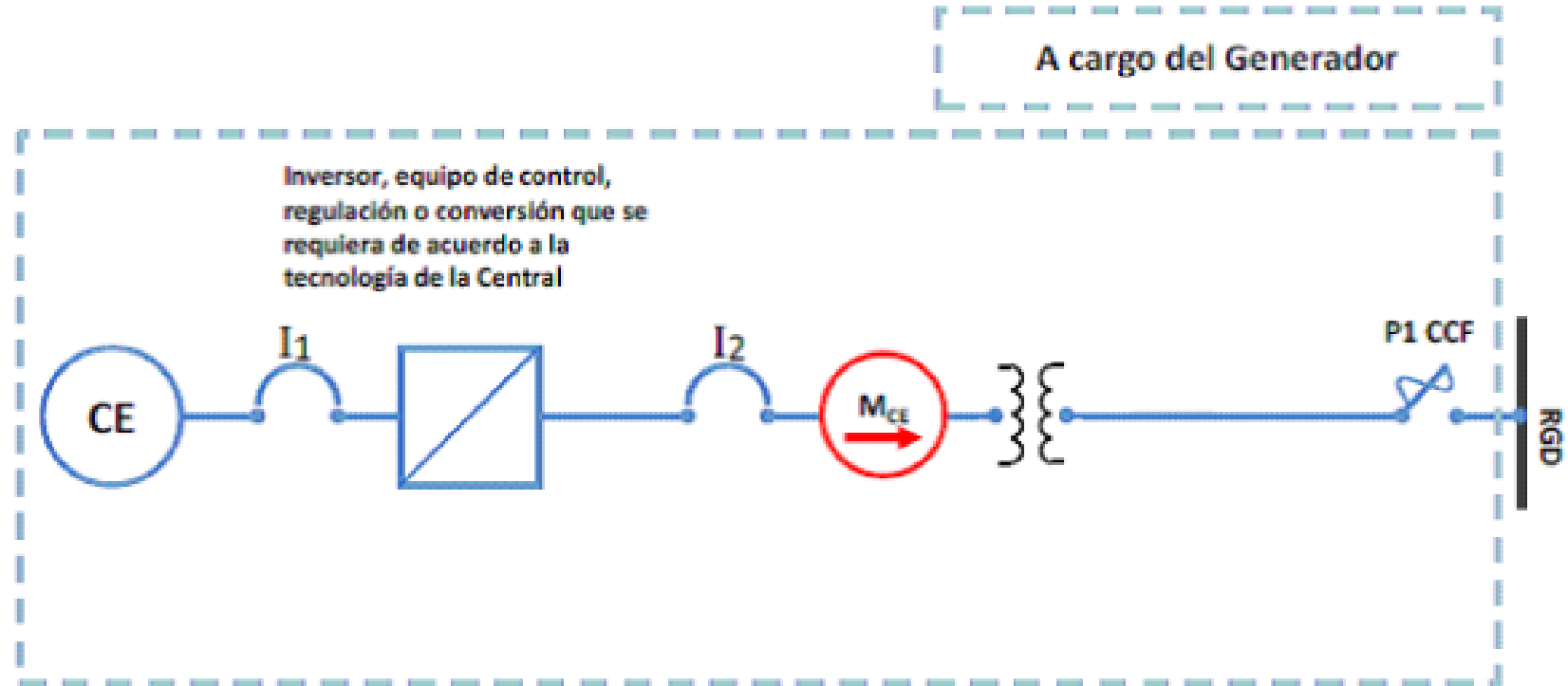
Esquema de interconexión 9 para Centrales Eléctricas mayores que 250 kW y menores que 500 kW en Media Tensión con medición en Media Tensión.
